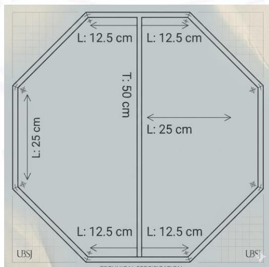
Gambar 6 : Detail Ukuran Papermob SEMOT 2026
